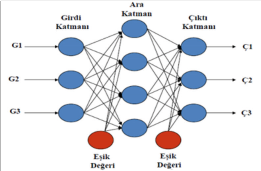
Görsel 3.18: Çok katmanlı algılayıcı modeli
